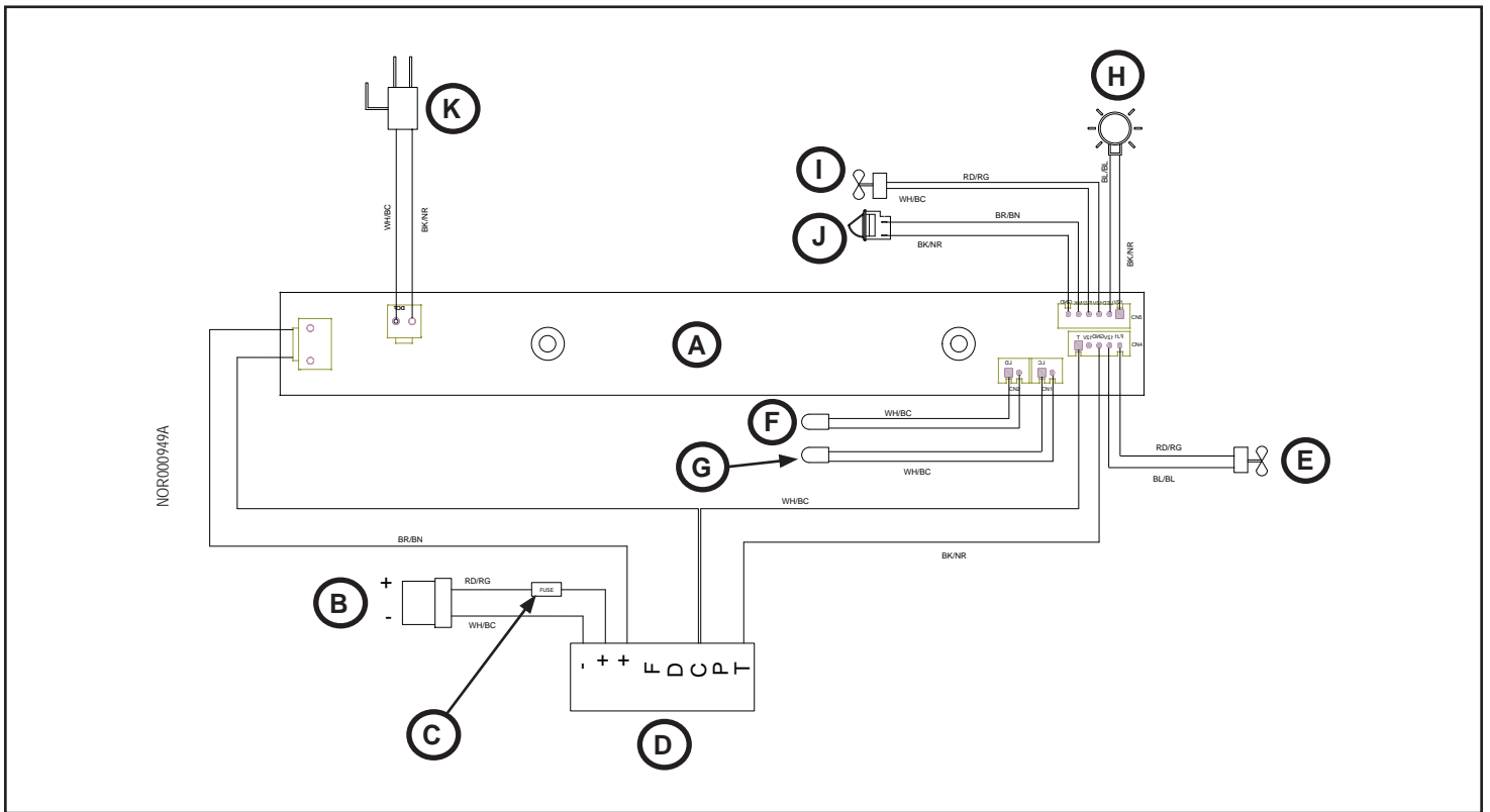
Fig. 6 - Wiring diagram
